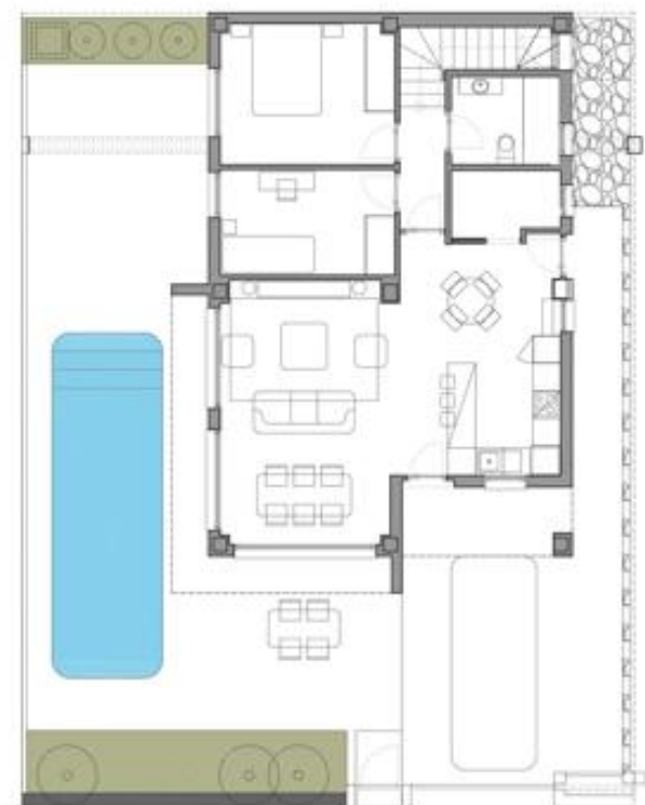
PLANTA BAJA
